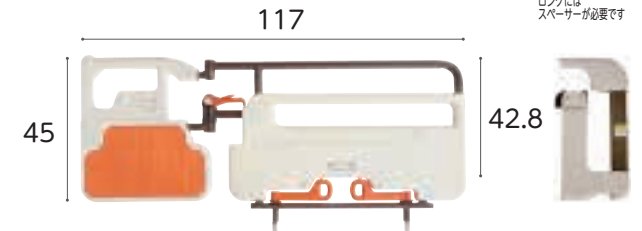
※アーム開閉角度: ± 135° (22.5° 刻み) ロングタイプ対応スペーサー (取付時サイズ幅 124 × 高さ 42.8)
